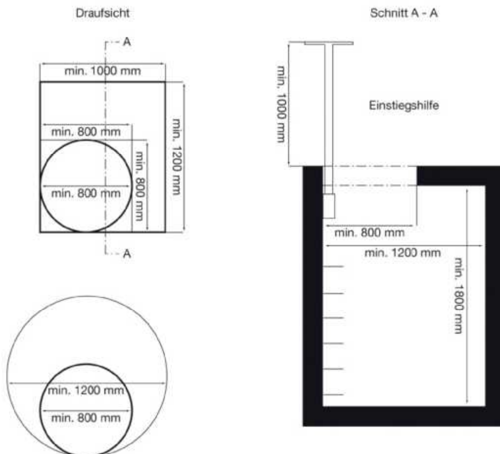
Bild 4: Schemazeichnungen begehbaren Wasserzählerschächte
