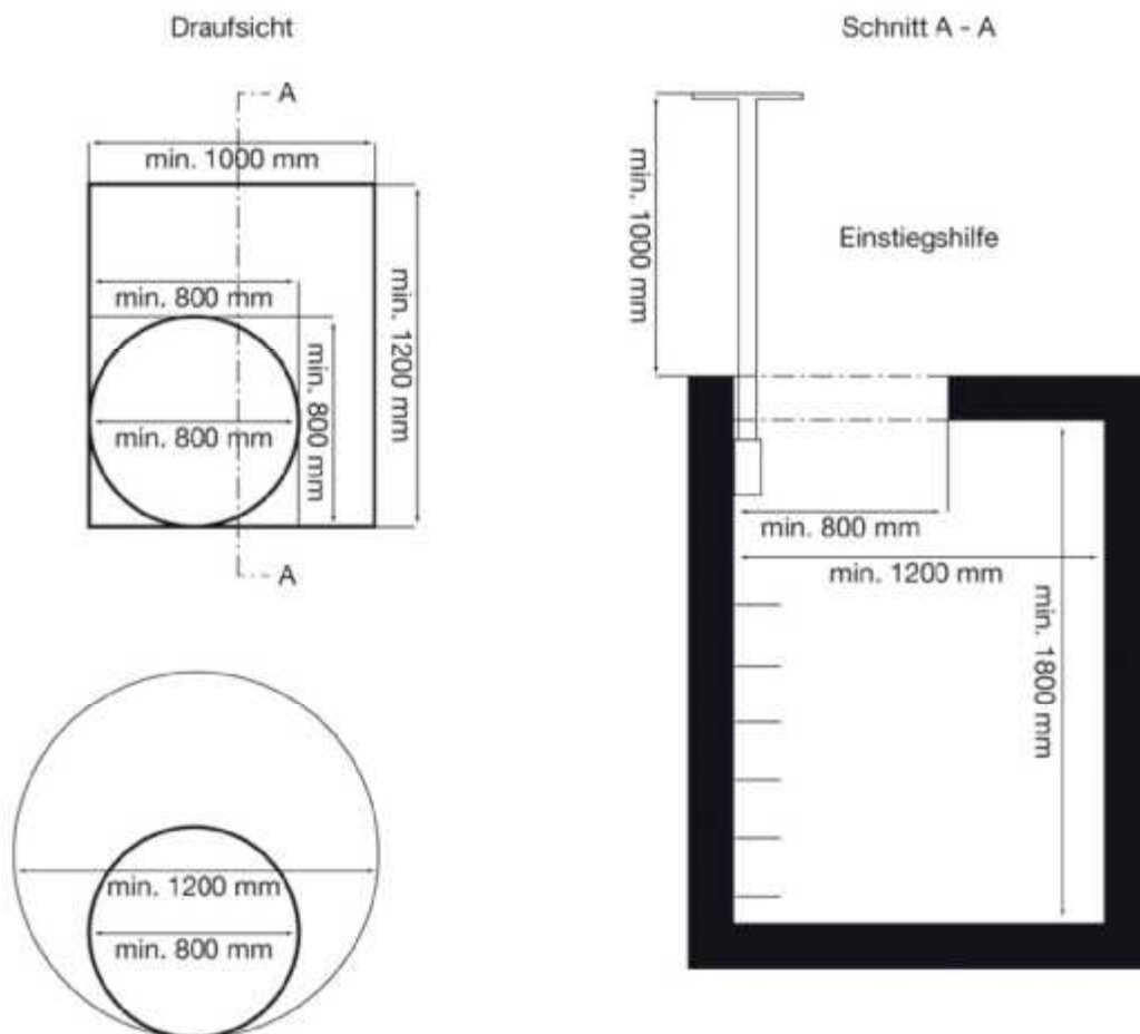
Bild 4: Schemazeichnungen begehbbarer Wasserzählerschächte
